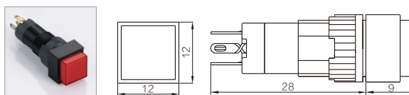
方形指示灯/按钮
