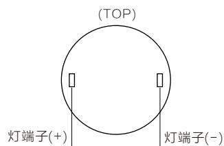
指示灯/ Indicator
