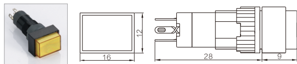
长方形指示灯/按钮
