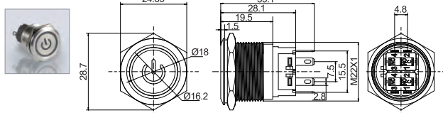
电源符号
