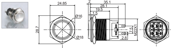
高面按钮
