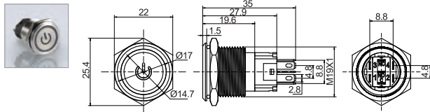
电源符号
