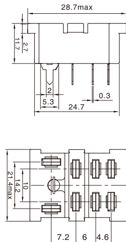
外形尺寸图 Dimensions
