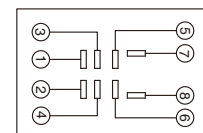
接线图 Wiring Diagram
