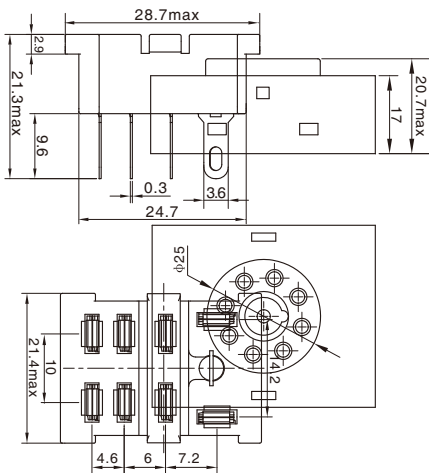
外形尺寸图 Dimensions
