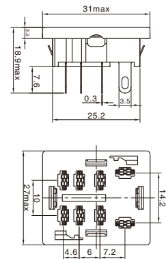
外形尺寸图 Dimensions
