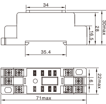
外形尺寸图 Dimensions
