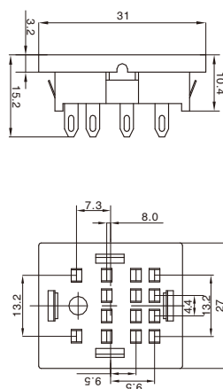
外形尺寸图 Dimensions
