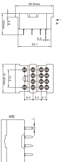
外形尺寸图 Dimensions
