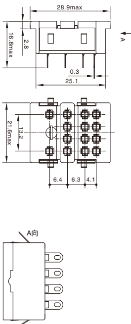
外形尺寸图 Dimensions
