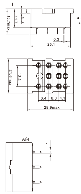
外形尺寸图 Dimensions
