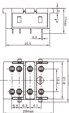
外形尺寸图 Dimensions
