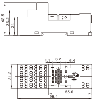
外形尺寸图 Dimensions
