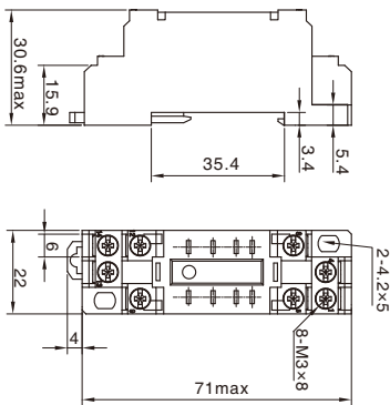
外形尺寸图 Dimensions
