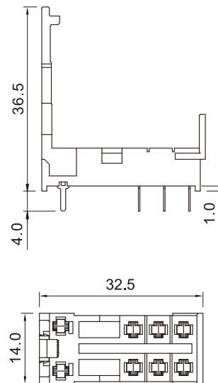
外形尺寸图 Dimensions
