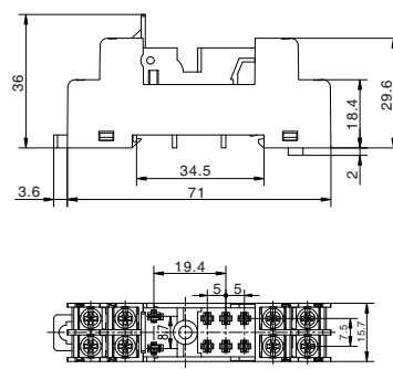
外形尺寸图 Dimensions
