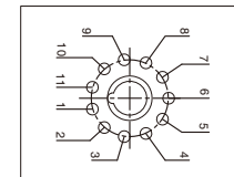
接线图 Wiring Diagram
