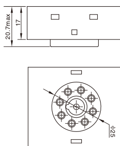
外形尺寸图 Dimensions
