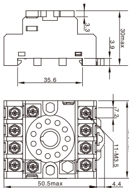
外形尺寸图 Dimensions
