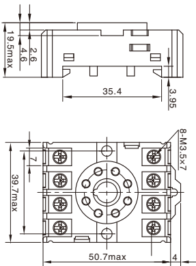
外形尺寸图 Dimensions
