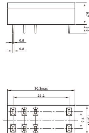
外形尺寸图 Dimensions
