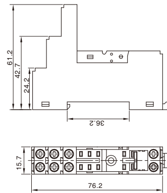
外形尺寸图 Dimensions
