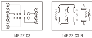
接线图 Wiring Diagram
