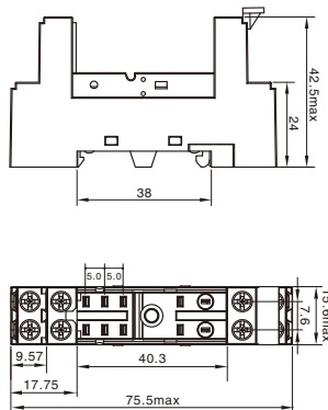
外形尺寸图 Dimensions
