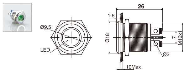
凹面信号灯螺丝型
