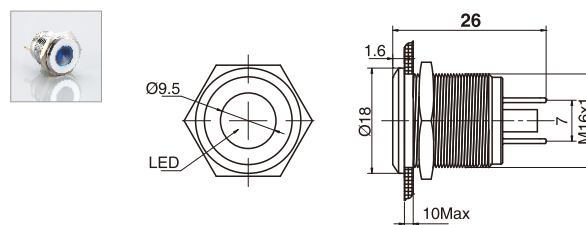
平面信号灯焊线型
