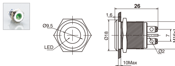
平面信号灯螺丝型
