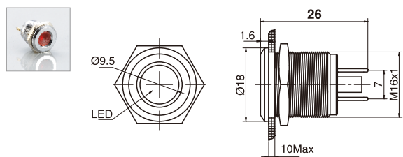
凹面信号灯焊线型
