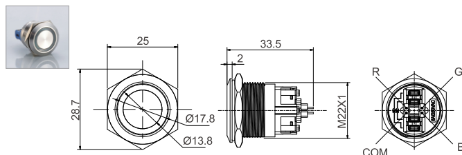
平面环形信号灯螺丝型
